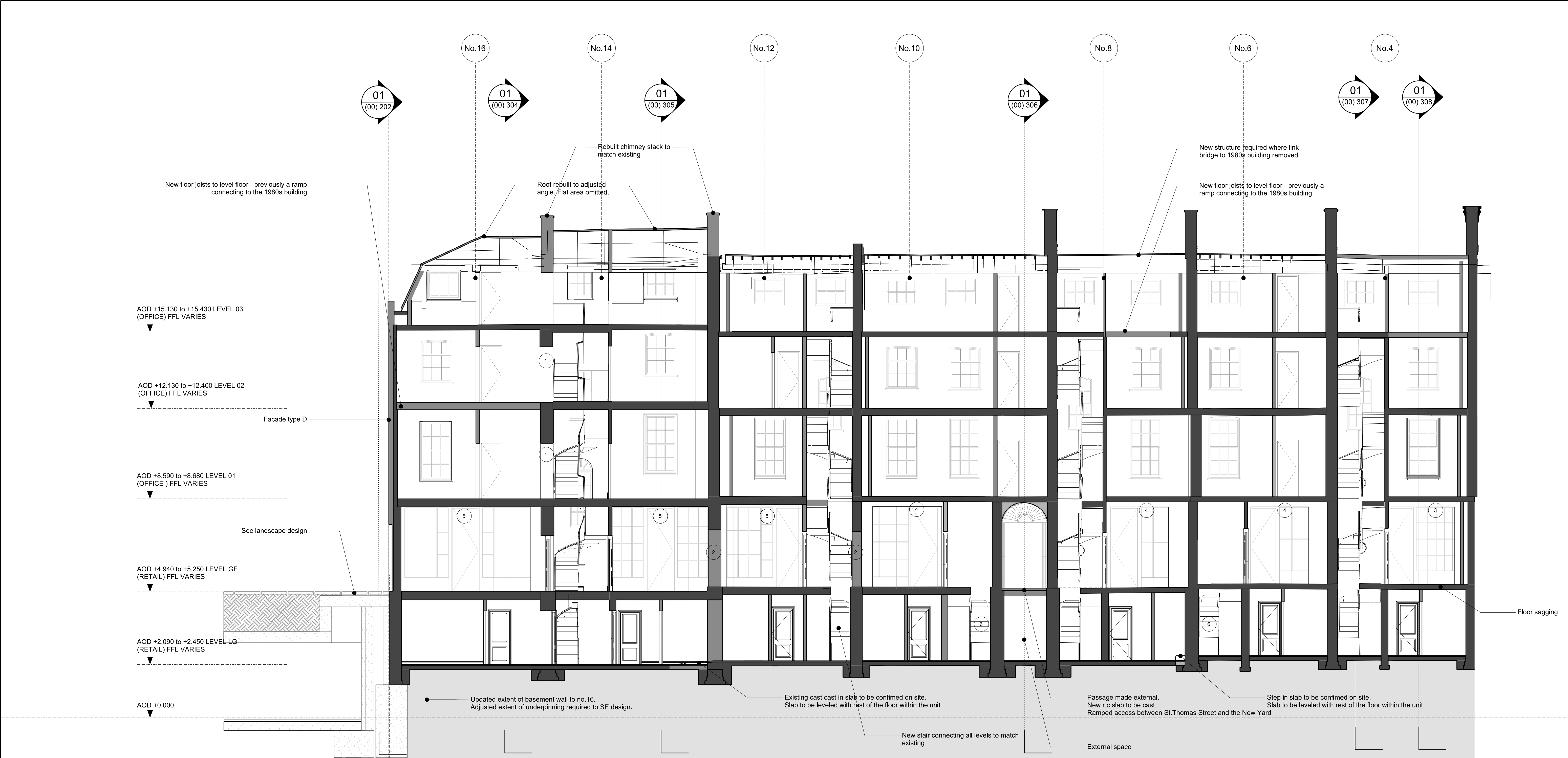
01 SECTION BB
